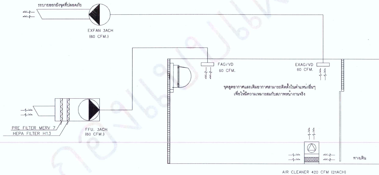
DIAGRAM ระบบปรับอากาศและระบายอากาศห้องทันตกรรม
